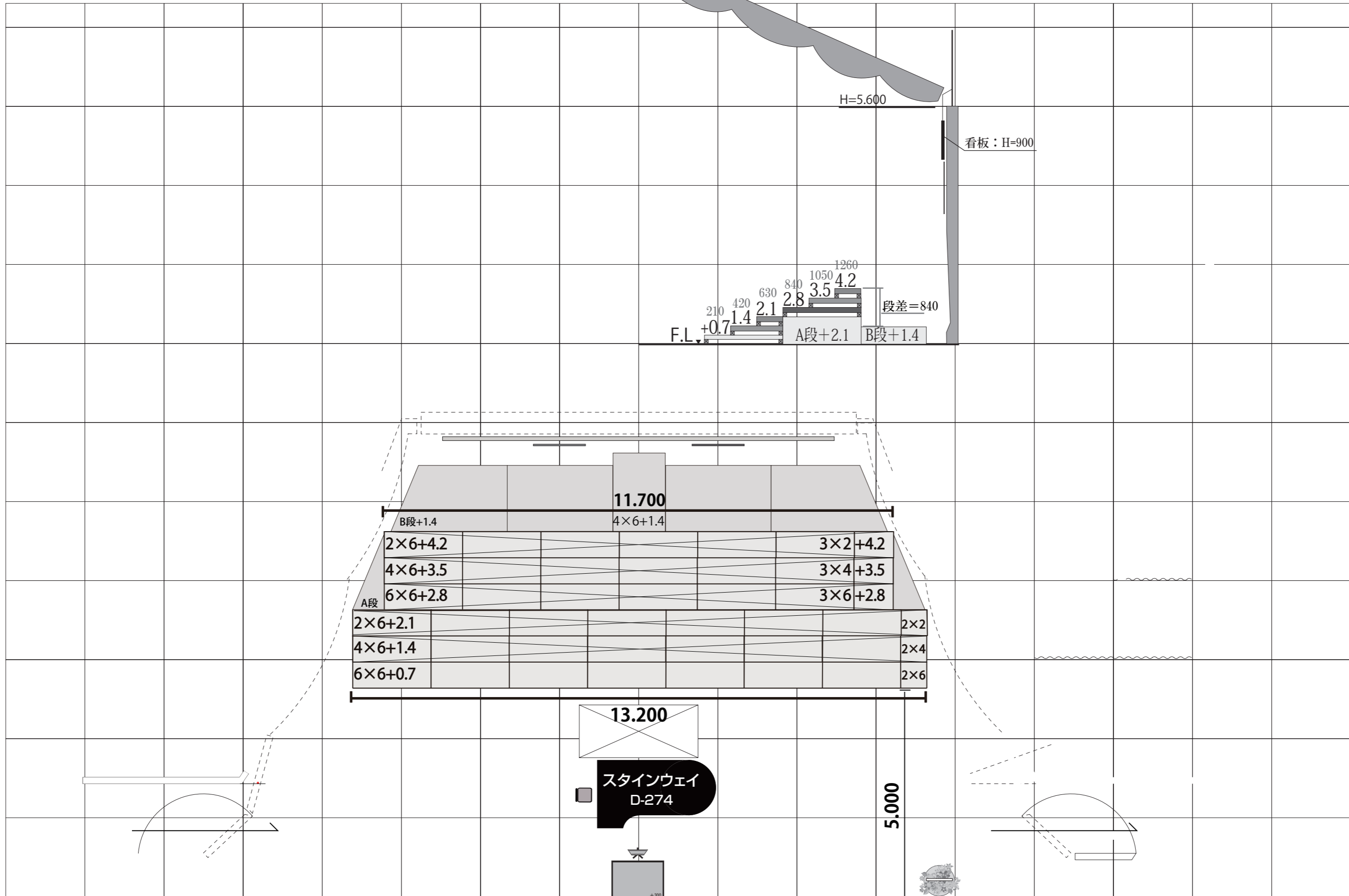
ホクト文化ホール(長野県民文化会館) 大ホール舞台平面図 方眼1目盛=1.818(1間)
